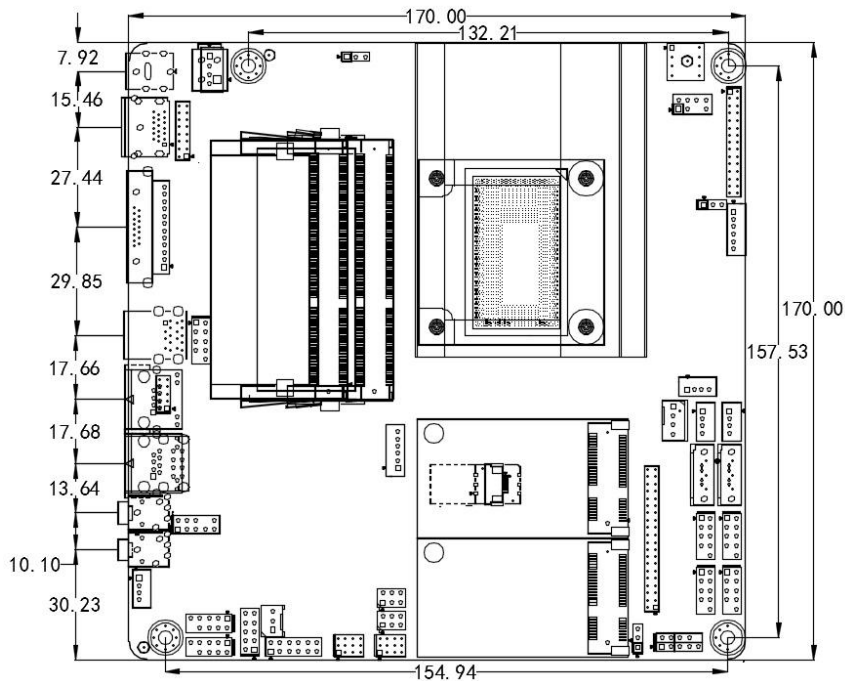
ITX-B670 VER:1.1尺寸图
