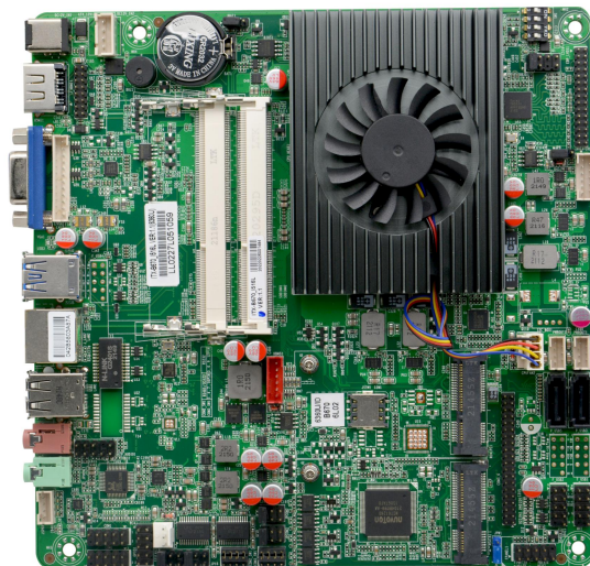
图一：ITX-B670 VER:1.1 主板正面图
