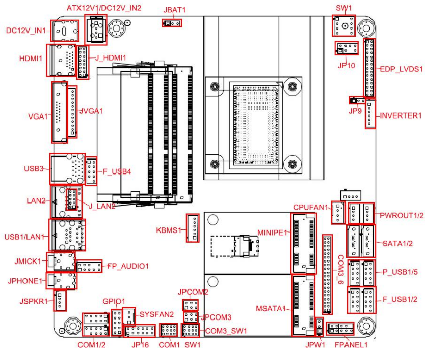
ITX-B670 接口位置图
