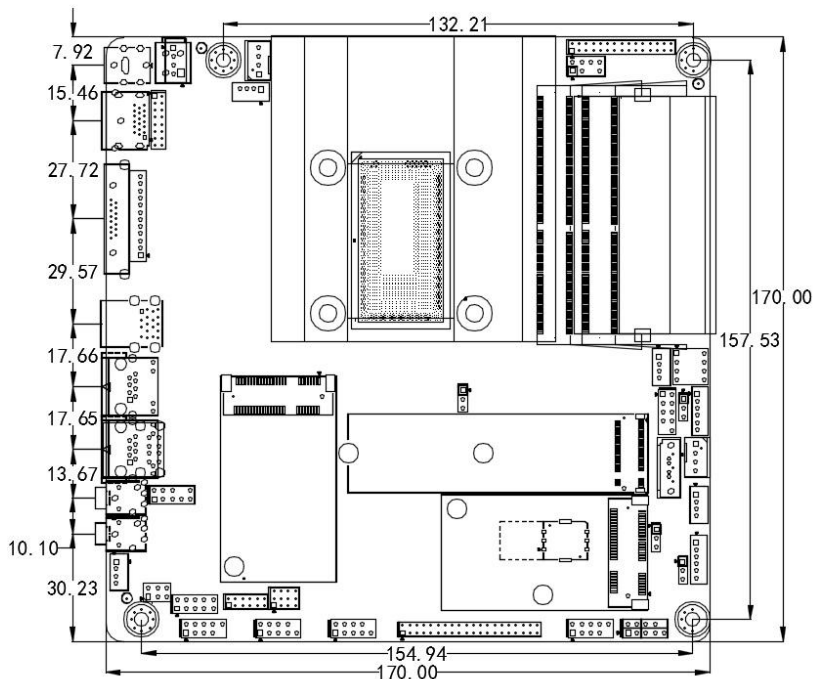
ITX-B100 VER:1.3尺寸图
