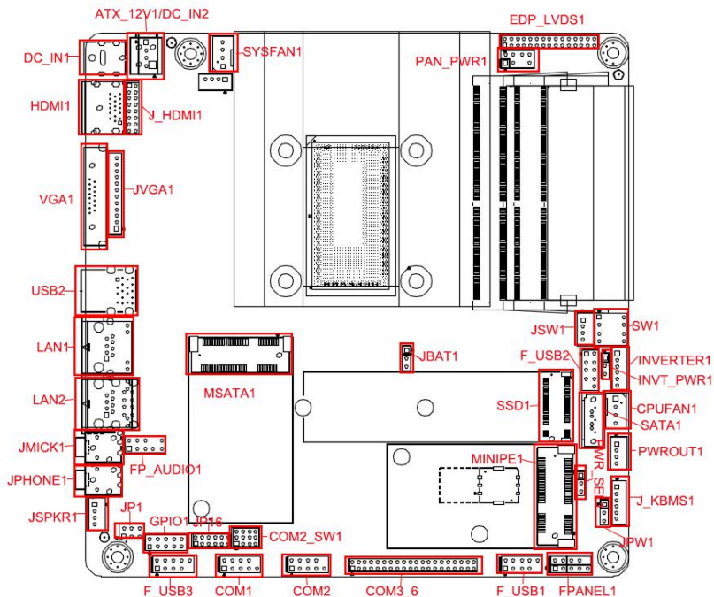
ITX-B100 接口位置图
