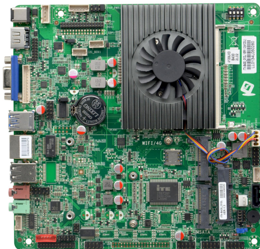
图一：ITX-B430_I312L VER:1.3 主板正面图
