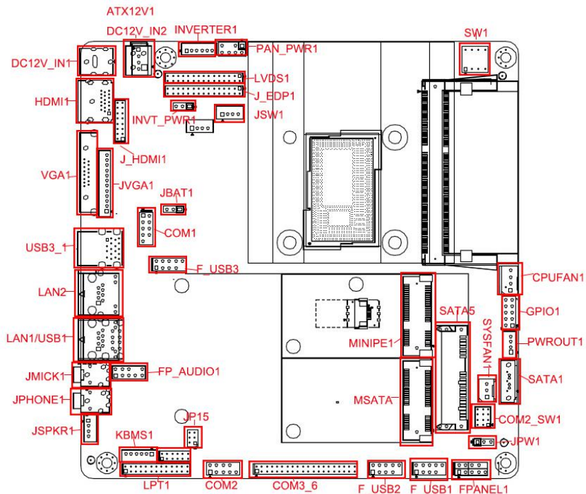
ITX-B430 VER:1.3 接口位置示意图
