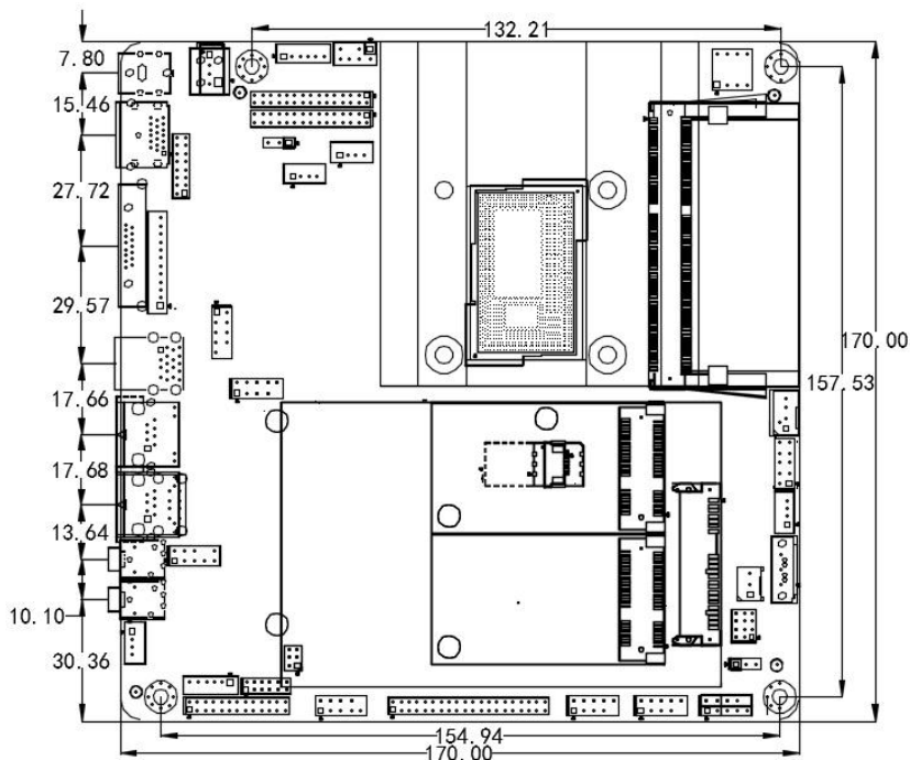
ITX-B430 VER:1.3 尺寸图
